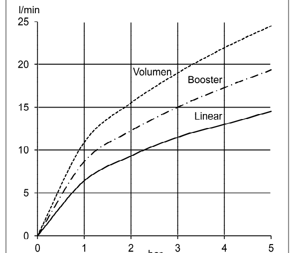
Durchflussdiagramm
