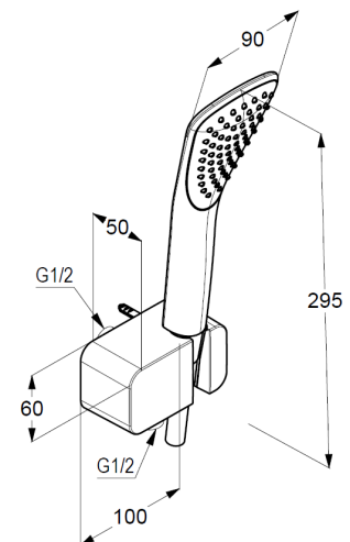
Maßzeichnung
