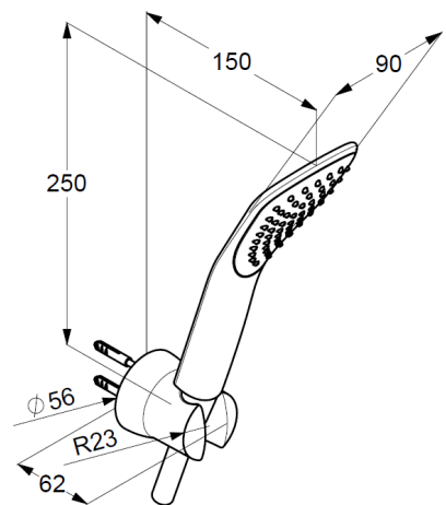
Maßzeichnung
