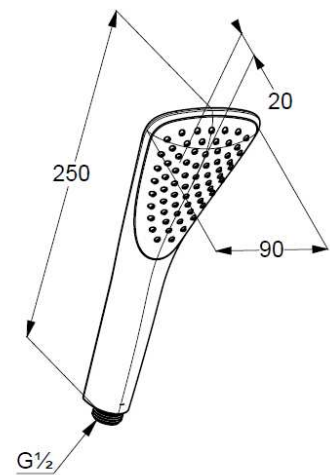
Maßzeichnung
