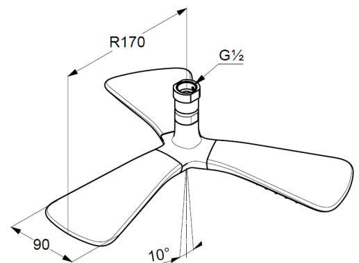
Maßzeichnung
