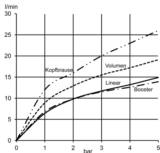
Durchflussdiagramm
