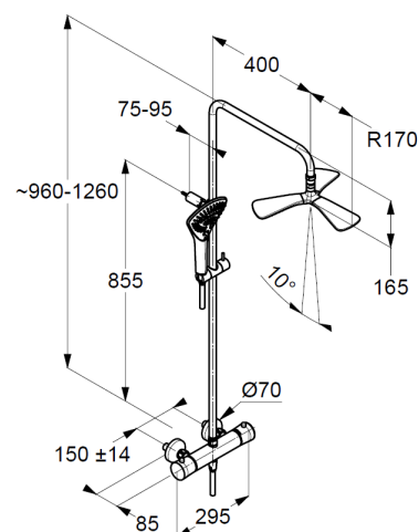
Maßzeichnung
