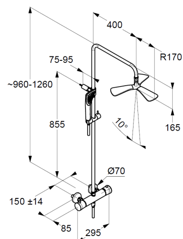
Maßzeichnung
