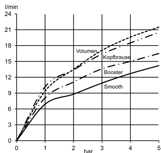
Durchflussdiagramm
