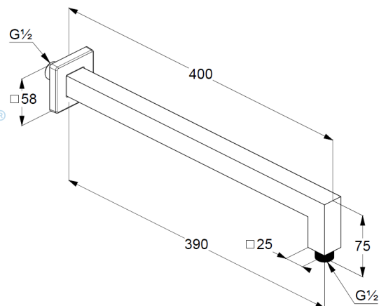
Maßzeichnung
