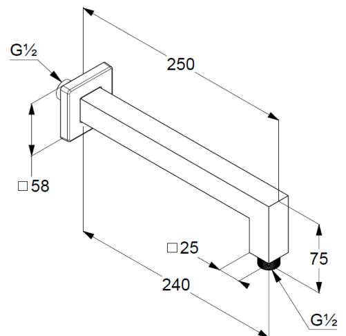
Maßzeichnung
