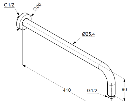
Maßzeichnung
