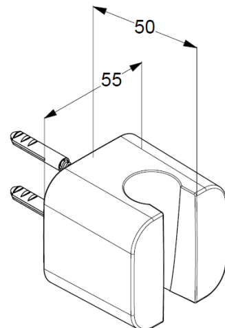
Maßzeichnung
