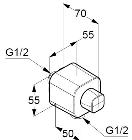
Maßzeichnung
