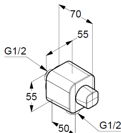
Maßzeichnung
