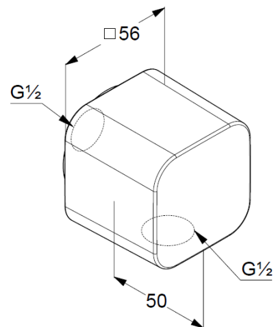
Maßzeichnung
