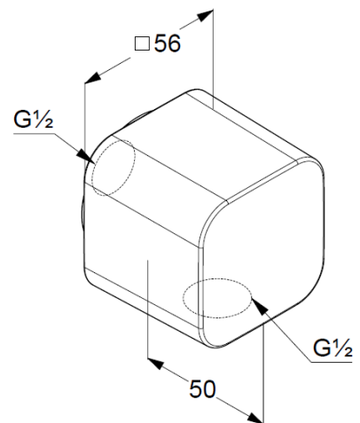
Maßzeichnung
