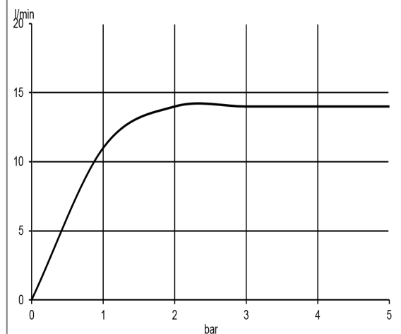
Durchflussdiagramm
