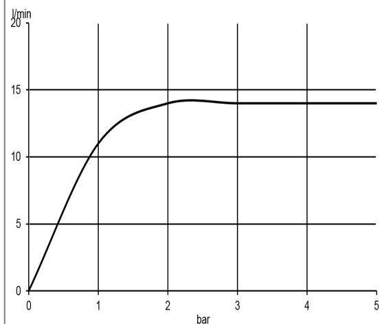
Durchflussdiagramm
