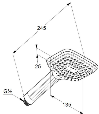
Maßzeichnung
