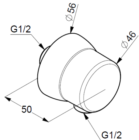
Maßzeichnung
