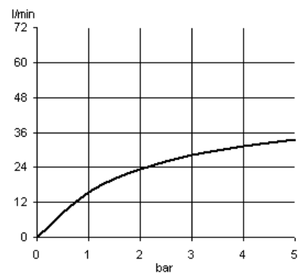
Durchflussdiagramm
