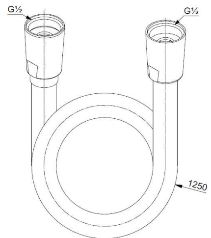
Maßzeichnung
