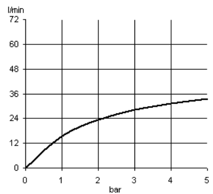
Durchflussdiagramm
