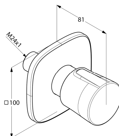
Maßzeichnung I
