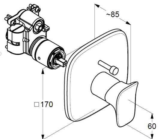
Maßzeichnung
