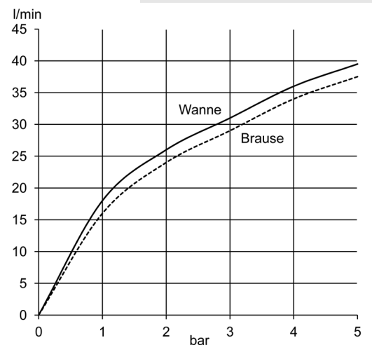
Durchflusssdiagramm
