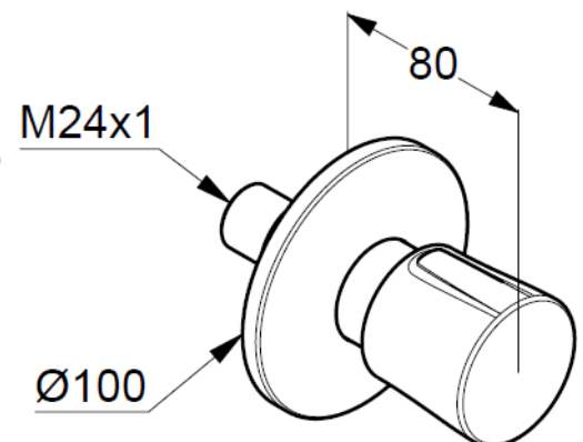
Maßzeichnung
