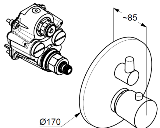
Maßzeichnung
