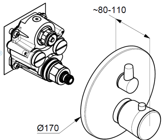
Maßzeichnung
