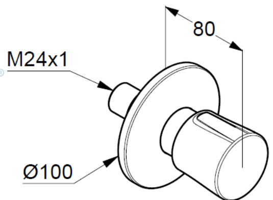
Maßzeichnung
