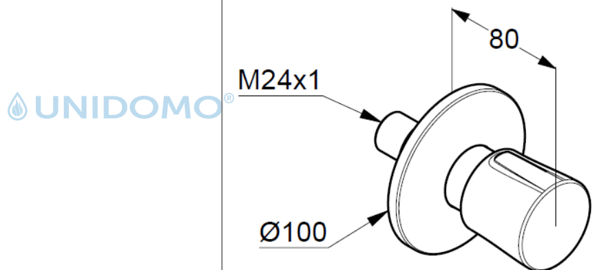
Maßzeichnung
