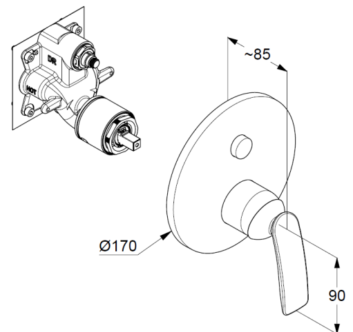
Maßzeichnung
