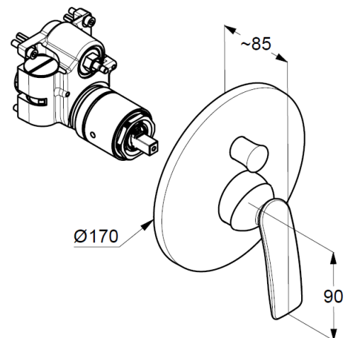
Maßzeichnung
