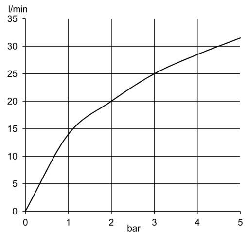
Durchflusssdiagramm
