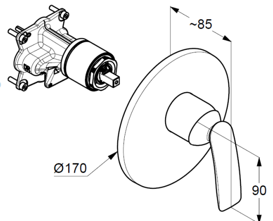
Maßzeichnung
