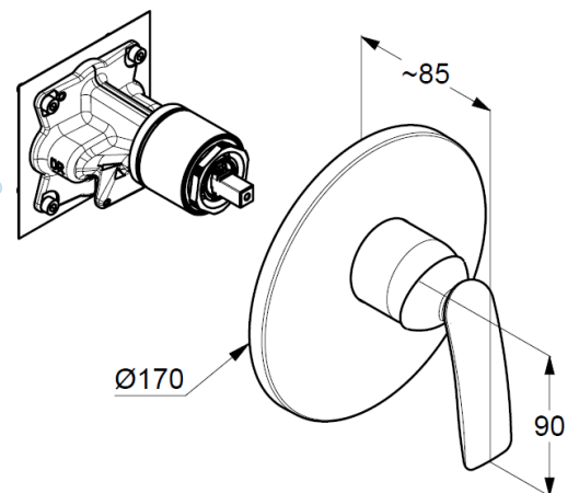
Maßzeichnung
