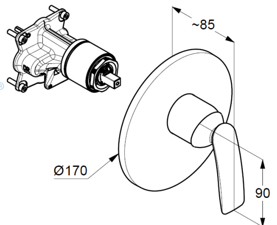
Maßzeichnung
