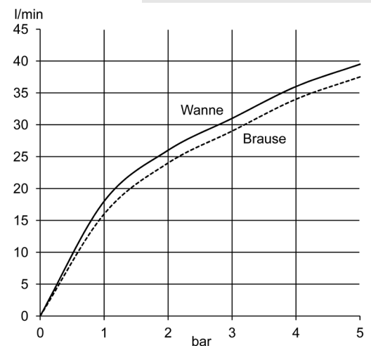
Durchflusssdiagramm
