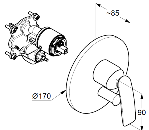
Maßzeichnung
