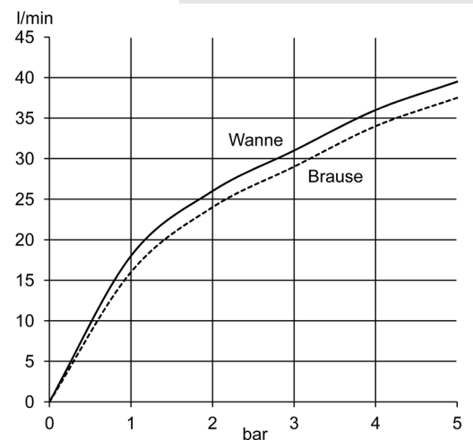
Durchflussdiagramm
