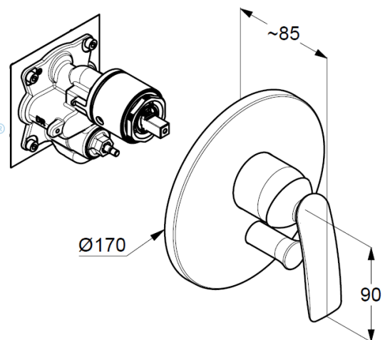
Maßzeichnung
