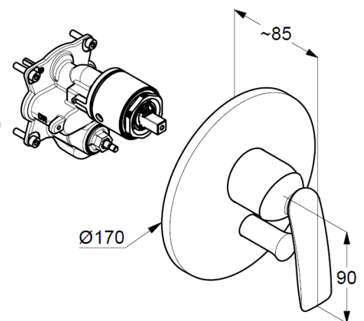
Maßzeichnung
