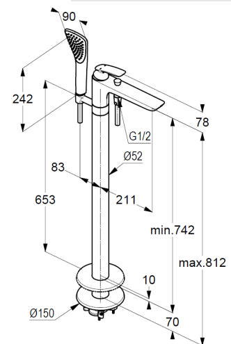
Maßzeichnung
