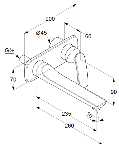
Maßzeichnung
