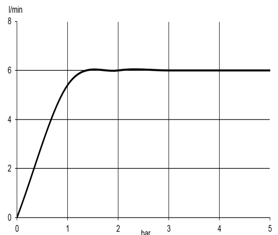
Durchflussdiagramm
