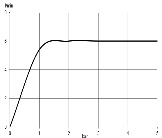
Durchflussdiagramm
