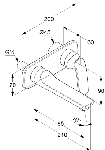
Maßzeichnung
