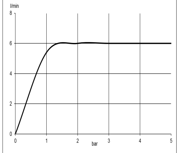
Durchflussdiagramm
