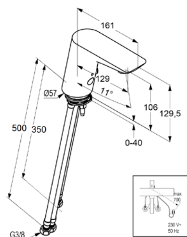
Maßzeichnung
