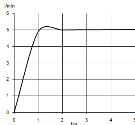
Durchflussdiagramm
