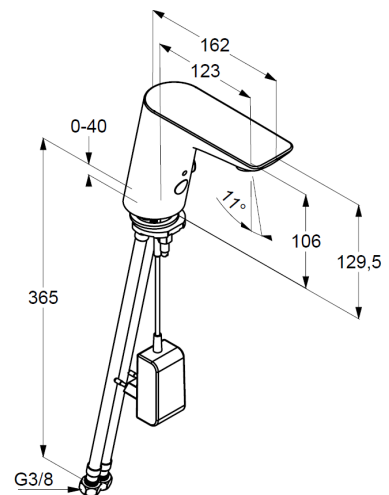
Maßzeichnung
