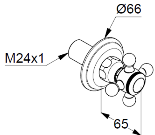
Maßzeichnung
