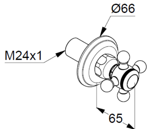
Maßzeichnung
