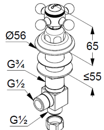
Maßzeichnung
