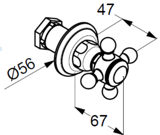
Maßzeichnung
