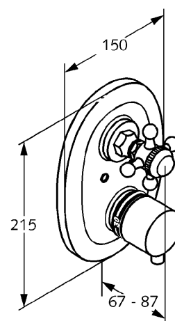
Maßzeichnung I
