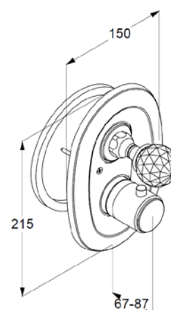
Maßzeichnung I
