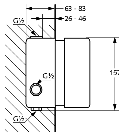
Maßzeichnung II
