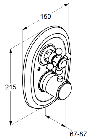
Maßzeichnung
